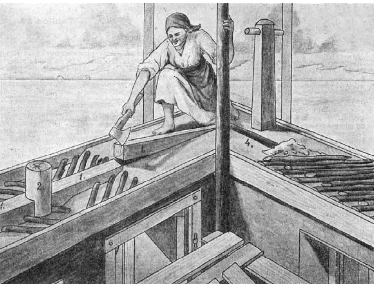
Ryc. 2. Wznoszenie ściany z gliny i chrustu opałowego, warstwowej z kanałami powietrznymi, według Mikołaja Niewierowicza (1930, s.57)
